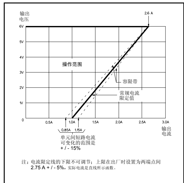
图 3 6V 电源的电流限制特性
